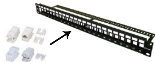
แผงกระจายสาย สามารถนำ Jack Outlet ตัวเมีย ทั้ง Cat.5e และ Cat.6 ใส่เข้าไปใน Frame เปล่า ได้ตามความเหมาะสม
